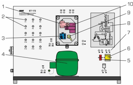
1 condensateur de service, 2 bobines-poussoirs des bornes, 3 relais de démarrage, 4 compresseur d'agent réfrigérant, 5 coupe-circuit automatique, 6 contacteur de puissance, 7 connecteurs de lecture, 8 schéma de connexion, 9 protection thermique, 10 condensateur de démarrage
